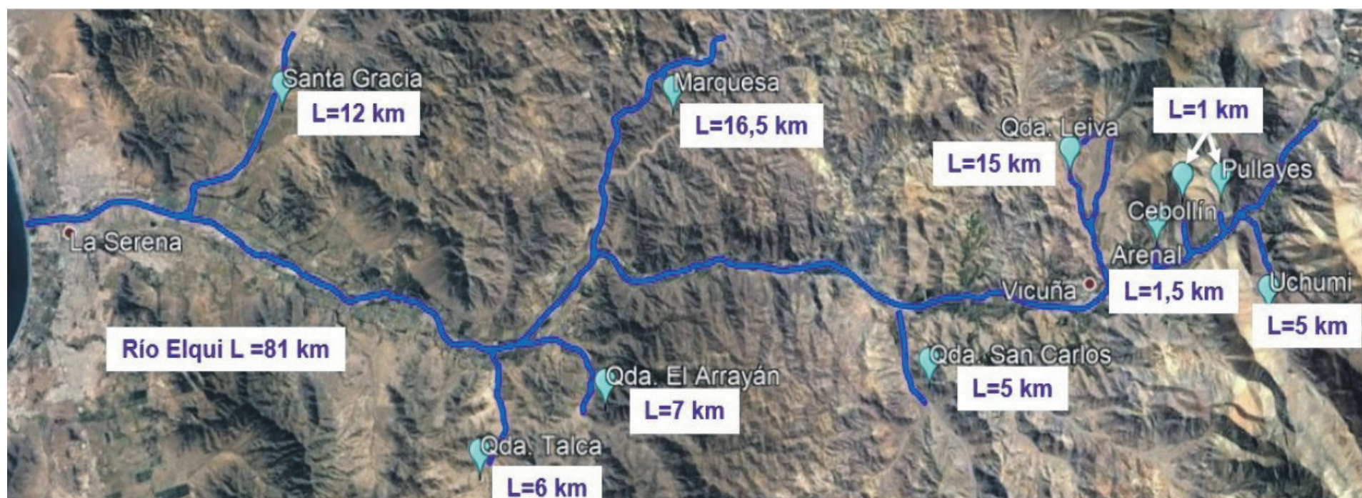
Este es el mapa de las quebradas que fueron estudiadas por el MOP. La simulación de inundación permitió identificar los puntos de mayor riesgo.
