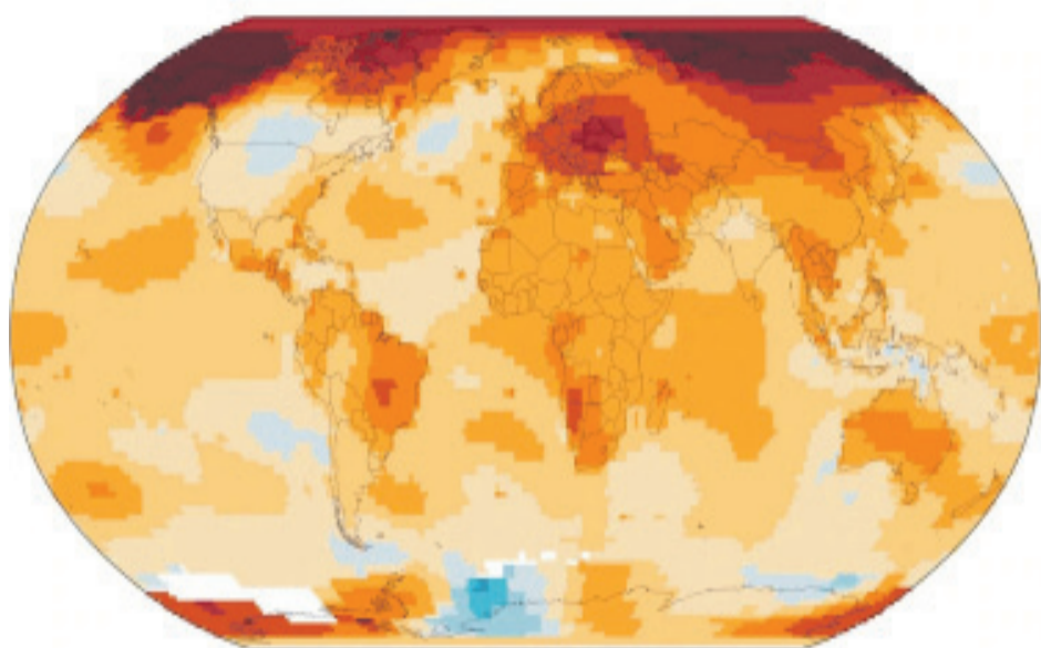
El calor en el planeta Tierra en 2019.
